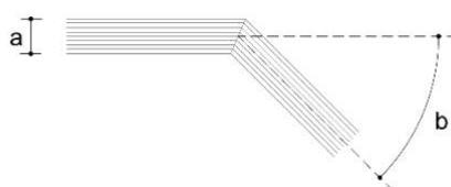
Ejemplo 41. Piezas en inglete de pavimento táctil indicador direccional señalizando cambios de dirección que formen un ángulo menor de 45° respecto del eje del sentido de la marcha.
