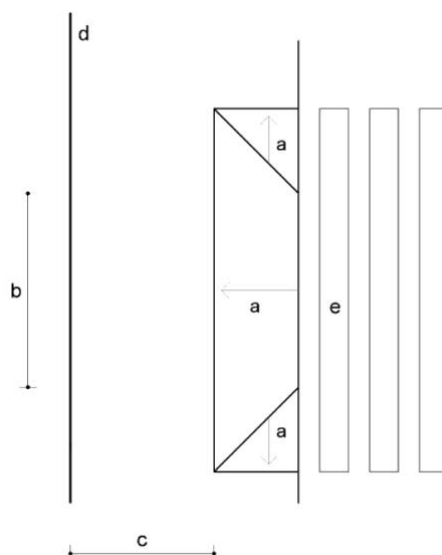
Ejemplo14. Esquema gráfico representando vado peatonal de tres planos inclinados.
