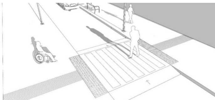
Ejemplo 37. Aplicación del pavimento táctil indicador en cruce con paso de peatones elevado.
